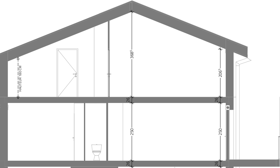
COUPE AA
